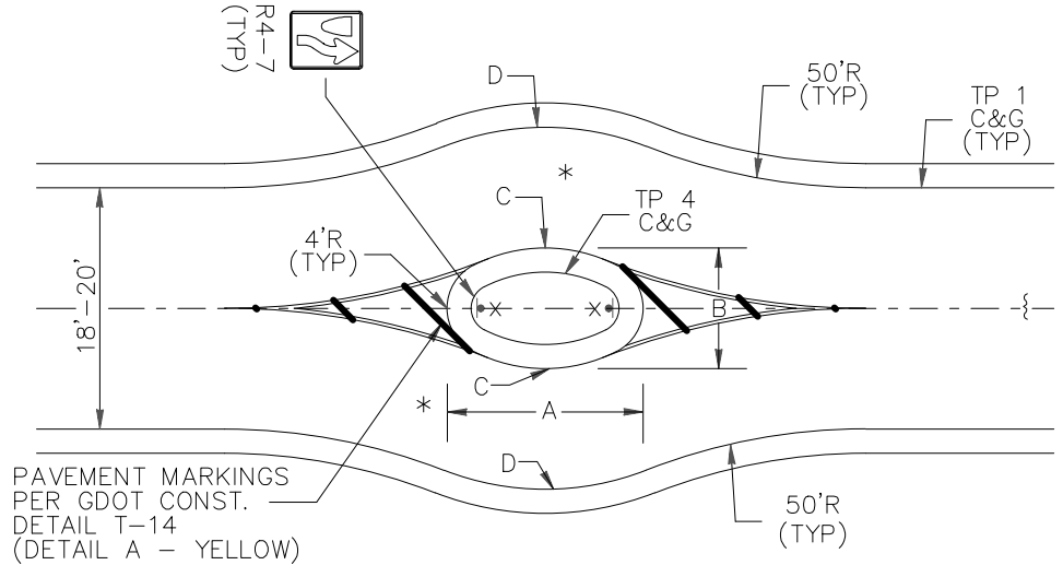
CENTER ISLAND 18-20' ROADWAY N.T.S.
